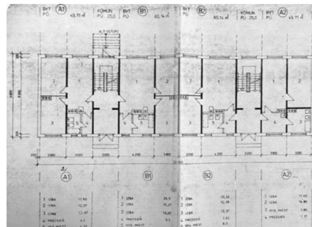
Obrázok 31 „Bytový dom pre cigánskych občanov P1.14 – PS Košice“ – pôdorys
